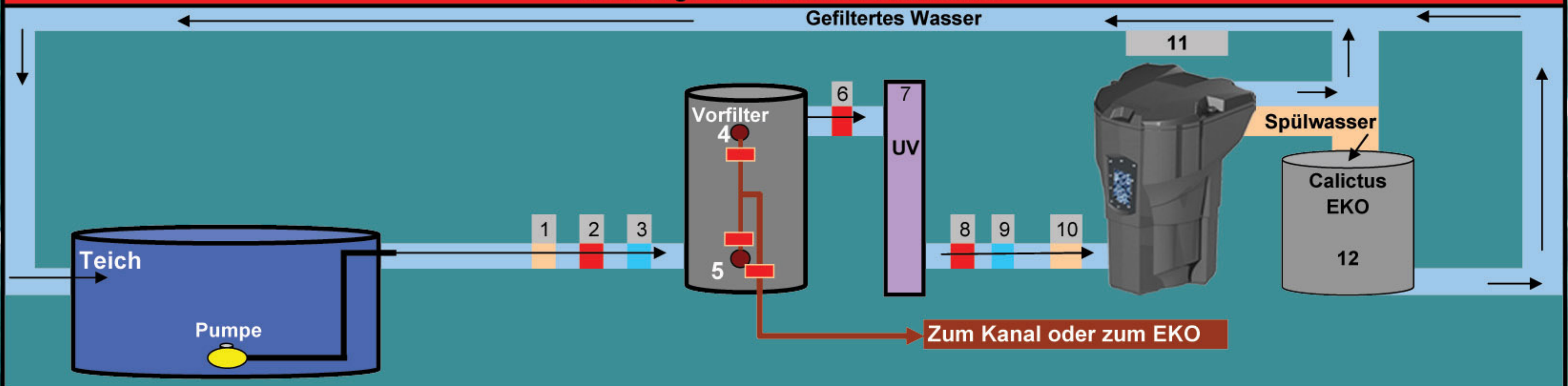
Zeichnung 2: Teich ohne Bodenablauf
